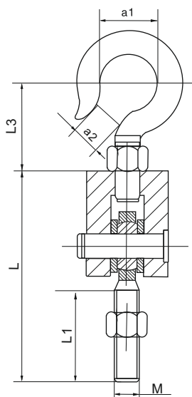
Монтажно-габаритные размеры мм (в дюймах)
